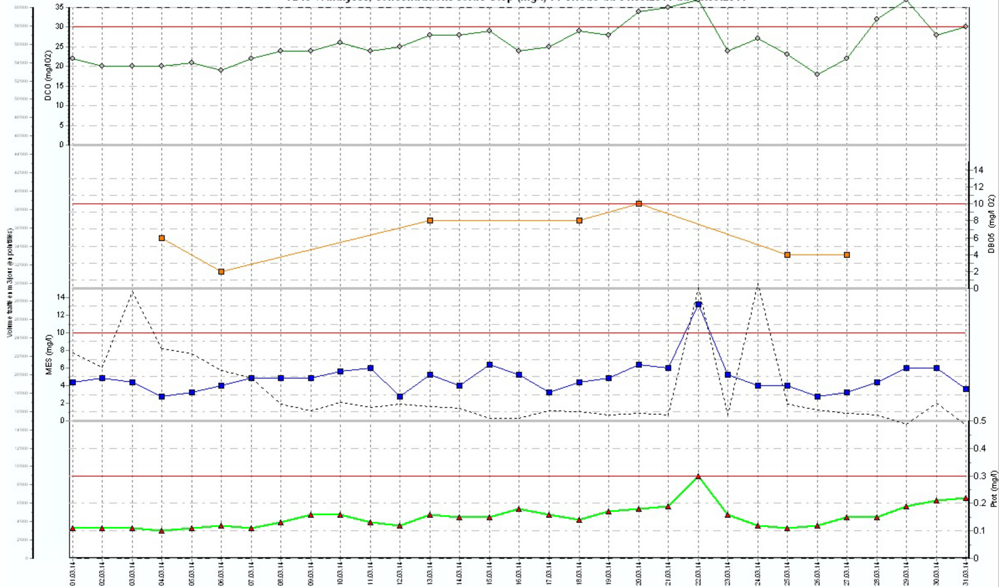
TB13 \ Analyses, concentrations sortie Step (mg/l) : Période du 01.03.2014 au 31.03.2014
