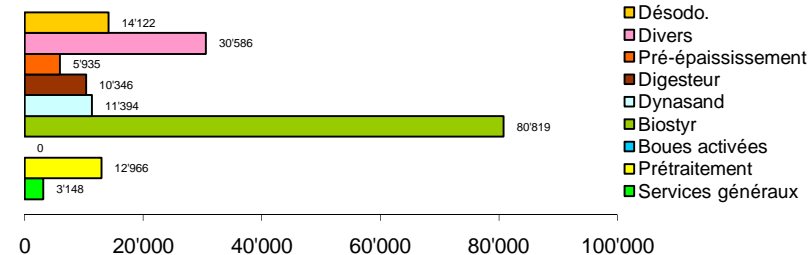
Répartition de la consommation d'électricité des différents process
