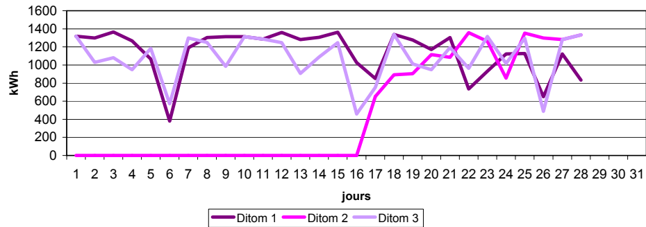
Evolution de la production électrique des moteurs à gaz
