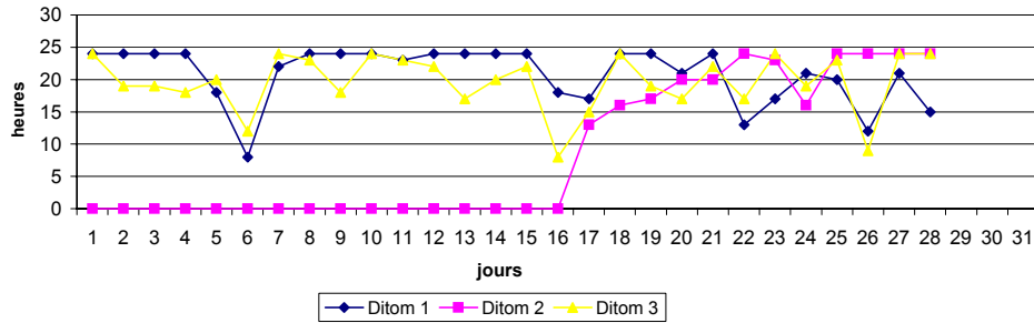
Evolution des temps de fonctionnement des moteurs à gaz
