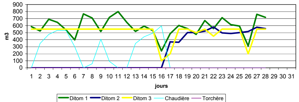
Evolution des volumes de gaz consommés
