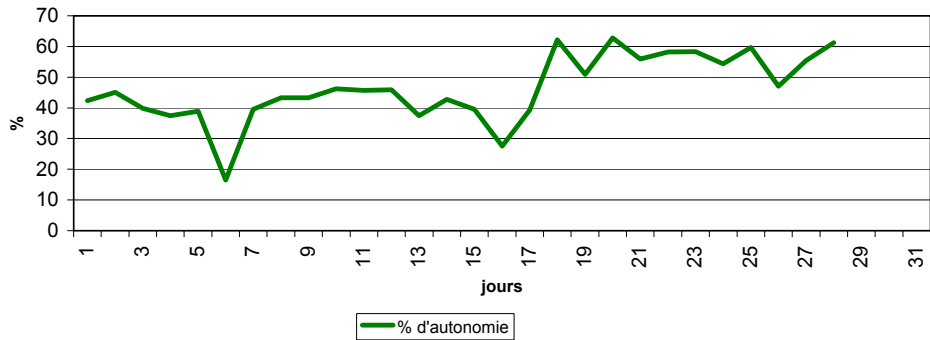
Evolution du taux d'autonomie électrique de la consommation de la step
