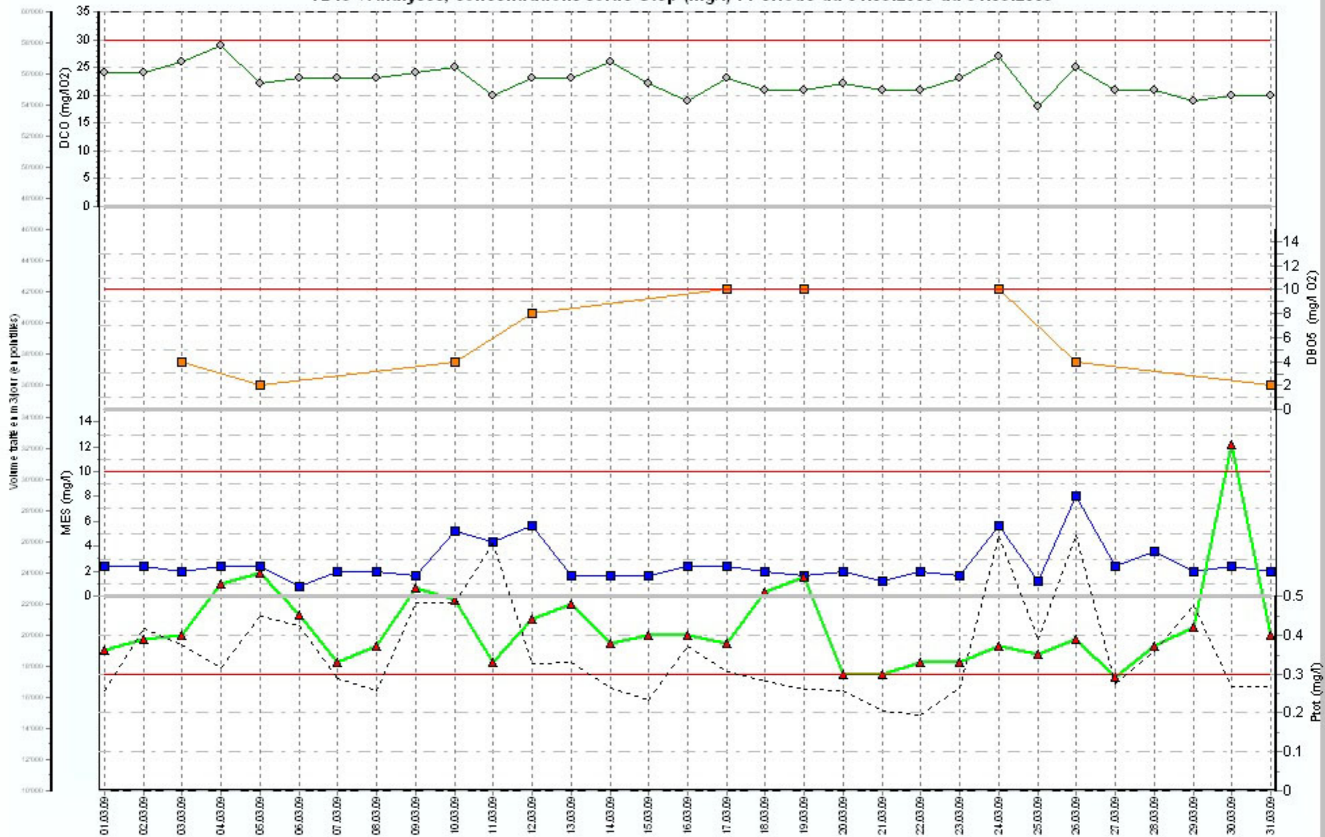
TB13 \ Analyses, concentrations sortie Step (mg/l) : Période du 01.03.2009 au 31.03.2009
