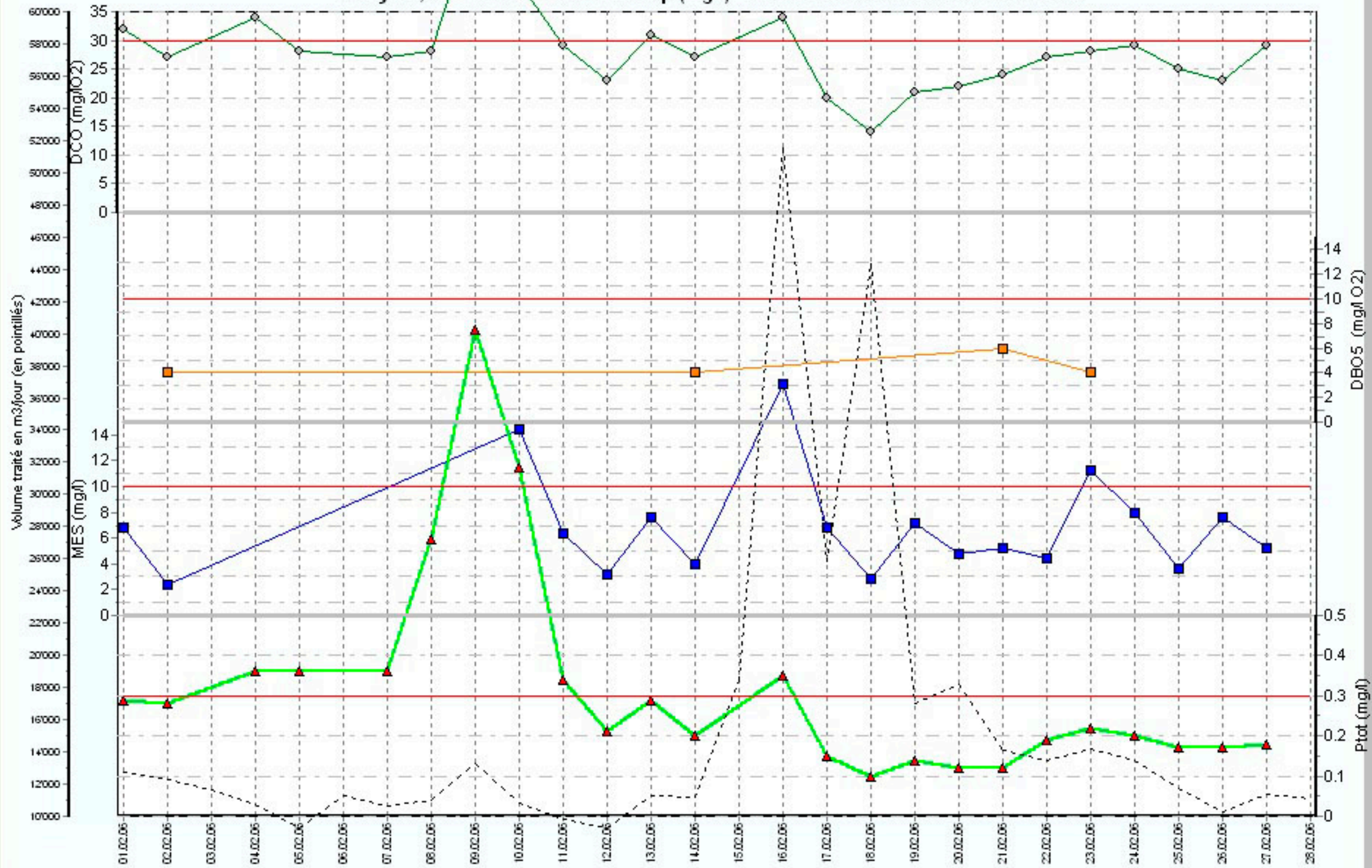
Analyses, concentrations sortie Step (mg/l) : Période du 01.02.2006 au 28.02.2006
